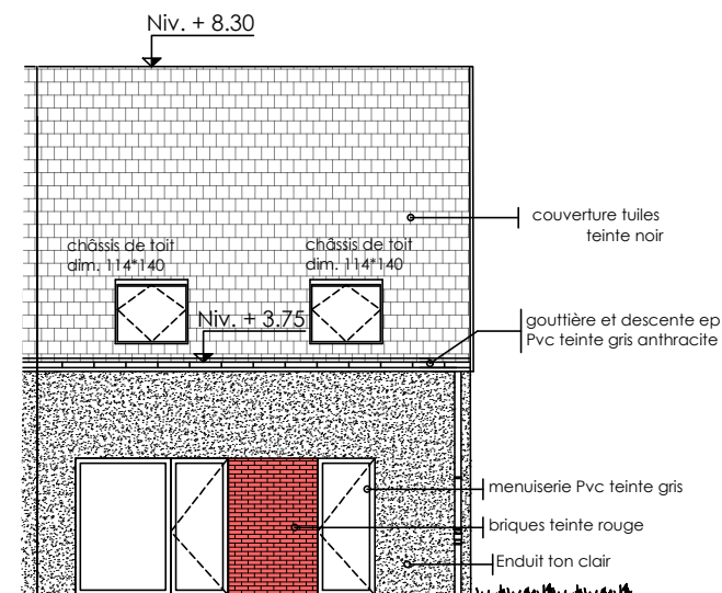
Façade Arrière
