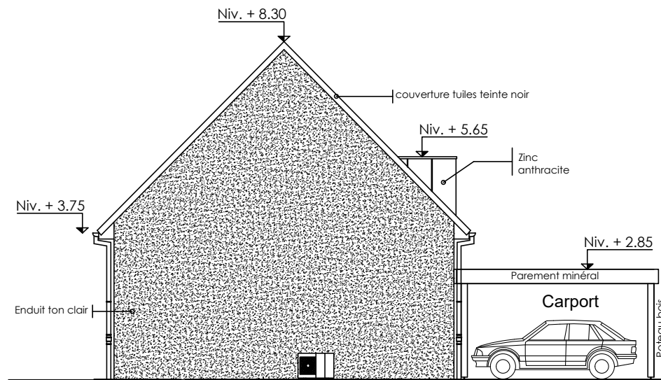
Pignon Gauche
